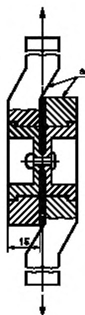
Рисунок 3 — Приспособление с установленной испытываемой заклепкой для разрешения спорного случая при испытании на срез
