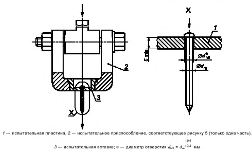
Рисунок 8 — Приспособление для испытания усилия разрыва сердечника
