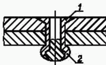
1 — головка «слепой» заклепки; 2 — «слепая» головка
