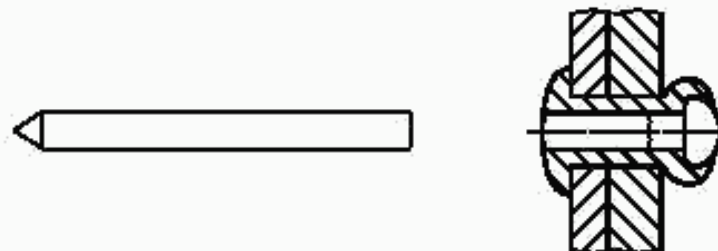
Рисунок 5 — Разрывающийся вытяжной сердечник
