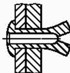
Рисунок 15 — Разделяющийся конец
