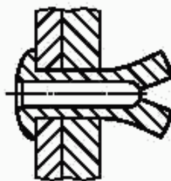
Рисунок 10 — Забивной штифт
