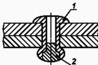
1 — головка «слепой» заклепки; 2 — «слепая» головка
