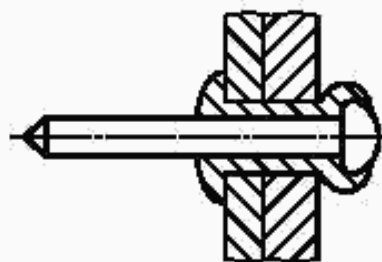
Рисунок 7 — Неразрывающийся вытяжной сердечник
