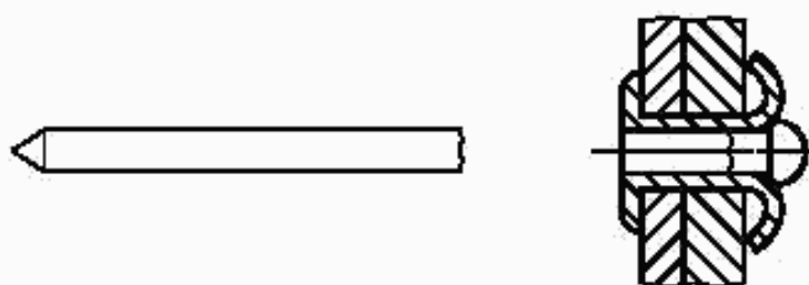
Рисунок 14 — Разделяющийся конец
