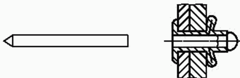
Рисунок 16 — Разрезной стержень
